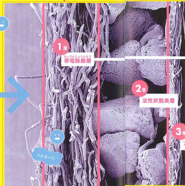
※Honda「アレルフリー高性能脱臭フィルター」断面の拡大写真(約35倍)
